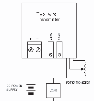
Wiring
